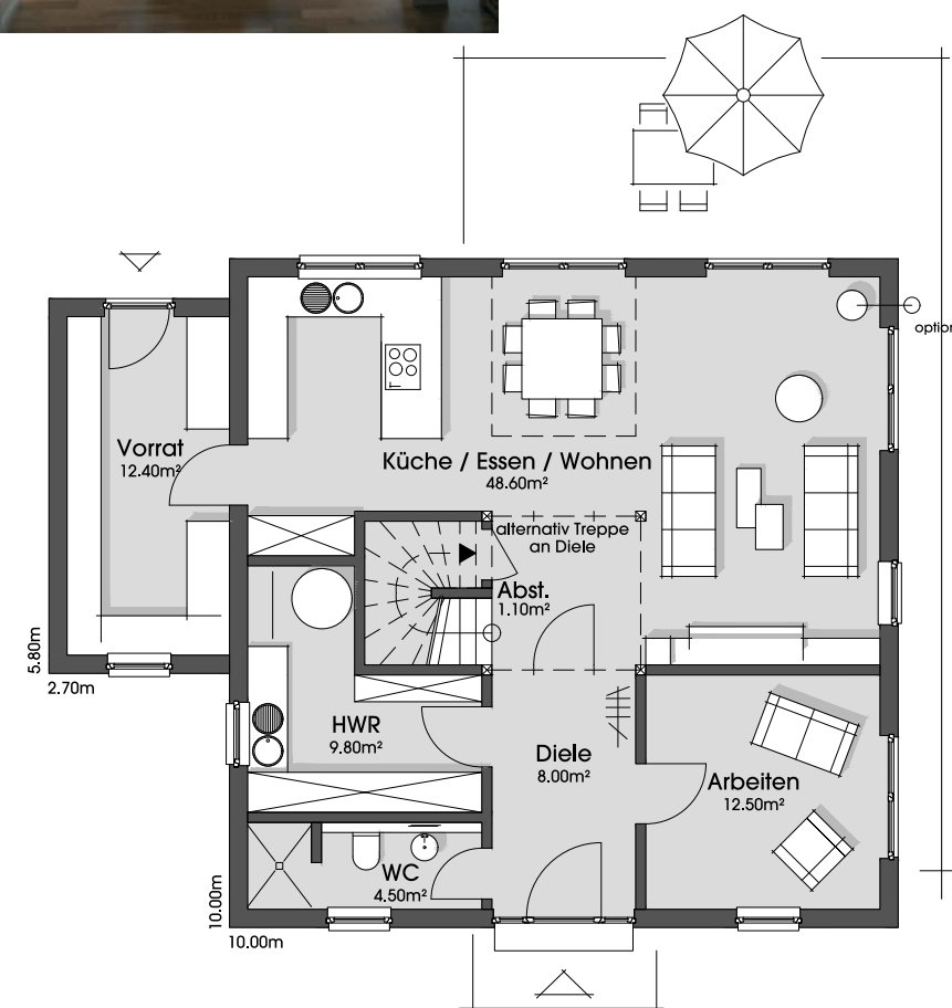
Erdgeschoss 1:125 95.80 m 2
