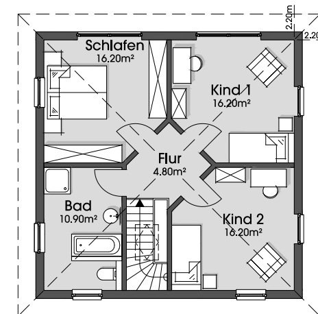
Dachgeschoss 1:175 64.30 m 2
