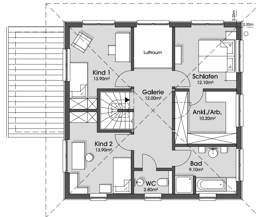
Obergeschoss 1:125 74.00m 2
